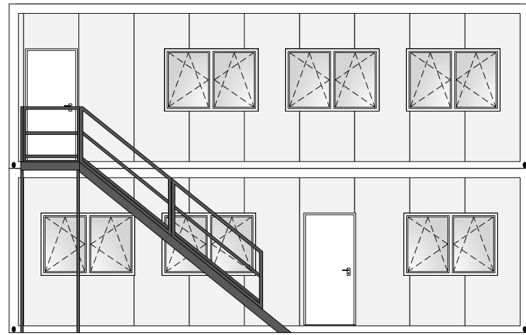
Voorgevel
