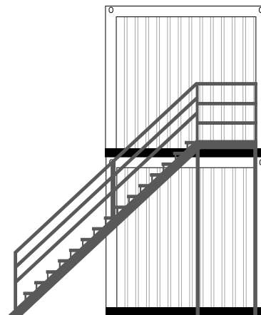
Rechter-aanzicht
