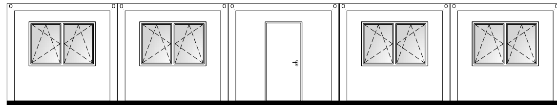
Voorgevel
